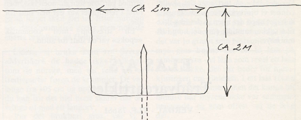
TVERRSNITT GJENNOM DYREGRAV. STEINMURTE SIDEKANTER KAN AV OG TIL FOREKOMME
